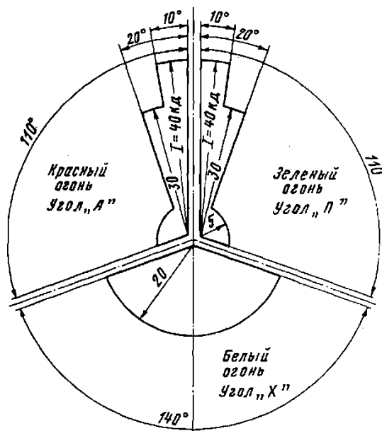
Рисунок 1387.1. - Светораспределение в горизонтальной плоскости для БАНО
