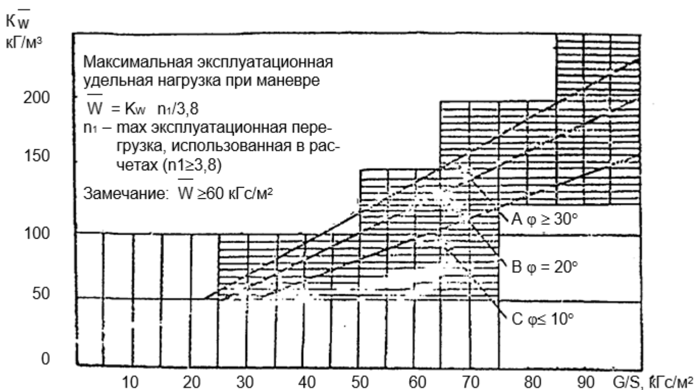
Рис. В1 МАКСИМАЛЬНАЯ ЭКСПЛУАТАЦИОННАЯ НАГРУЗКА НА ПОВЕРХНОСТИ ОПЕРЕНИЯ ПРИ МАНЕВРЕ В ЗАВИСИМОСТИ ОТ УГЛА ОТКЛОНЕНИЯ
