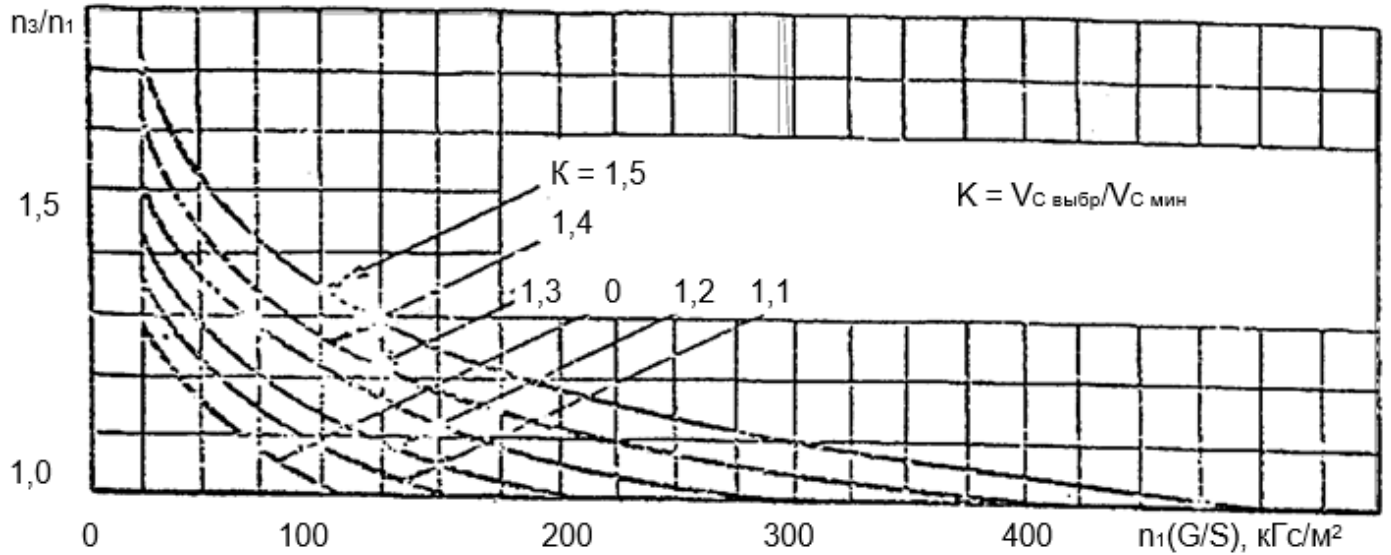
Рис. А1 ГРАФИКИ ДЛЯ ОПРЕДЕЛЕНИЯ ЗНАЧЕНИЙ p_3 В ЗАВИСИМОСТИ ОТ ЗНАЧЕНИЯ V_c
