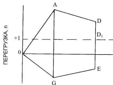
Рис. 2. Маневры в вертикальной плоскости
