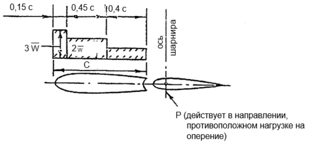
Рис. В6 РАСПРЕДЕЛЕНИЕ ВОЗДУШНОЙ НАГРУЗКИ НА СТАБИЛИЗИРУЮЩИХ ПОВЕРХНОСТЯХ ХВОСТОВОГО ОПЕРЕНИЯ
