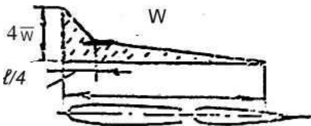
Рис. В8 РАСПРЕДЕЛЕНИЕ ВОЗДУШНОЙ НАГРУЗКИ НА ПОВЕРХНОСТЬ ХВОСТОВОГО ОПЕРЕНИЯ
