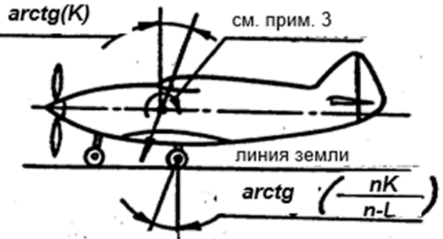
Горизонтальная посадка с носовым колесом находящимся в непосредственной близости у земли
