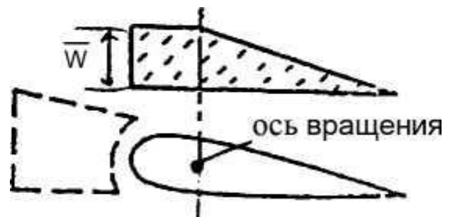
Рис. В9 РАСПРЕДЕЛЕНИЕ ВОЗДУШНОЙ НАГРУЗКИ НА ЭЛЕРОНЕ
