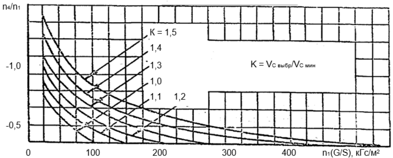
Рис. А2 ГРАФИКИ ДЛЯ ОПРЕДЕЛЕНИЯ ЗНАЧЕНИЙ p_4 В ЗАВИСИМОСТИ ОТ ЗНАЧЕНИЯ V_c
