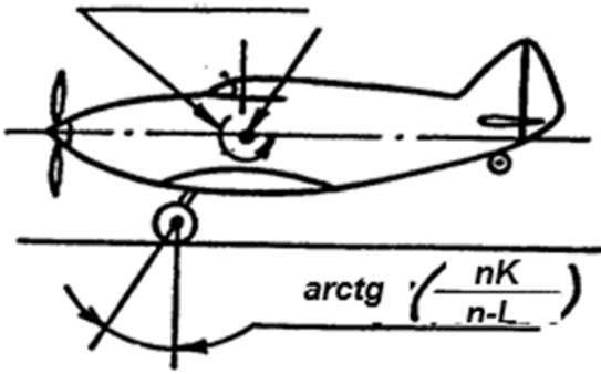
Горизонтальная посадка
