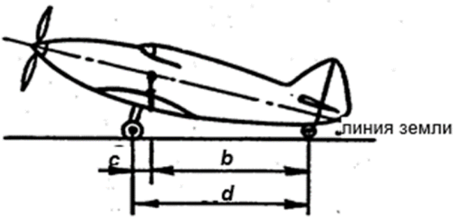
Посадка на 3 точки с опущенной хвостовой опорой
