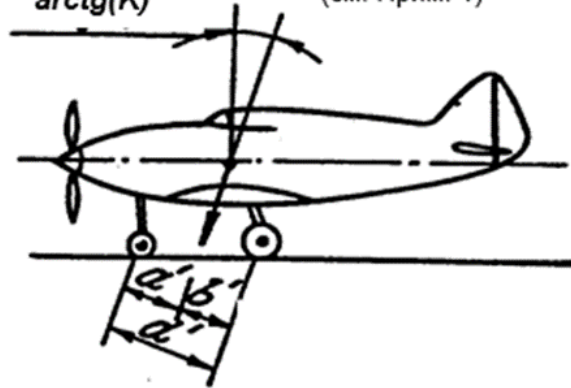
Горизонтальная посадка с реакциями земли, направленными под углом
