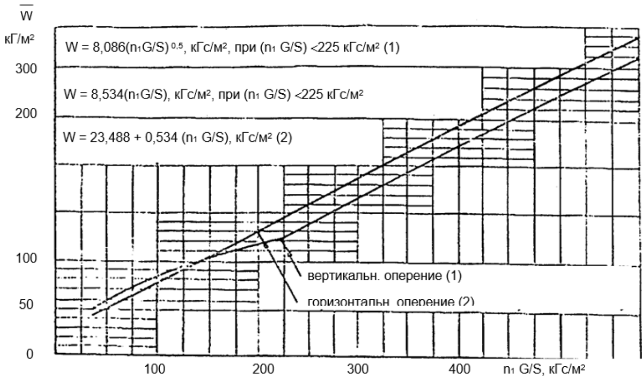
Рис. А4 РАСЧЕТ УДЕЛЬНОЙ НАГРУЗКИ ПРИ МАНЕВРЕ НА ОПЕРЕНИЕ
